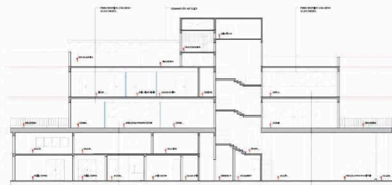
2 CORTE BB ESCALA 1:100
