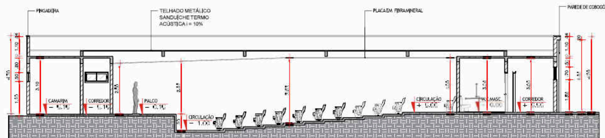
1 CORTE AA" ESCALA 1/75
