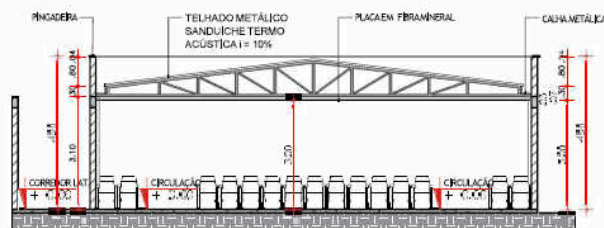
2 CORTE BB" ESCALA 1/75
